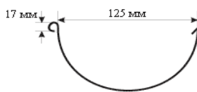
Сечение желоба
