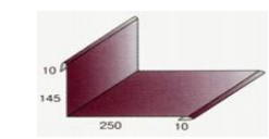
Планка примыкания верхняя
