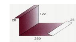
Планка примыкания нижняя
