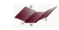
Ендова верхняя
