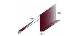
Планка снегозадержателя
